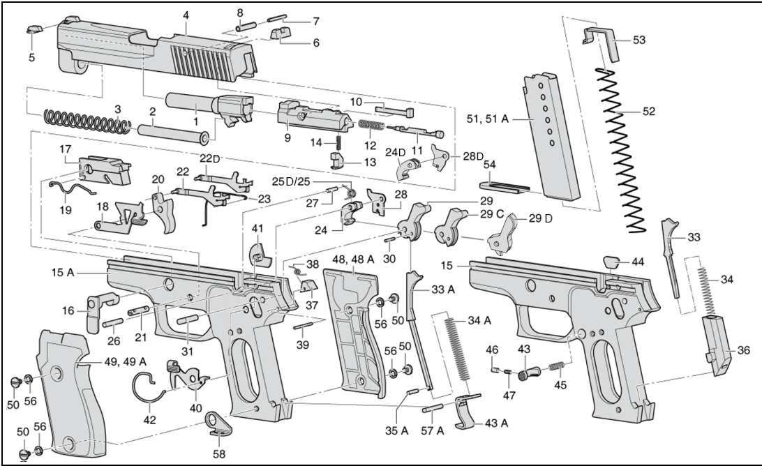
Abb. 17, Ersatzteile P 220
