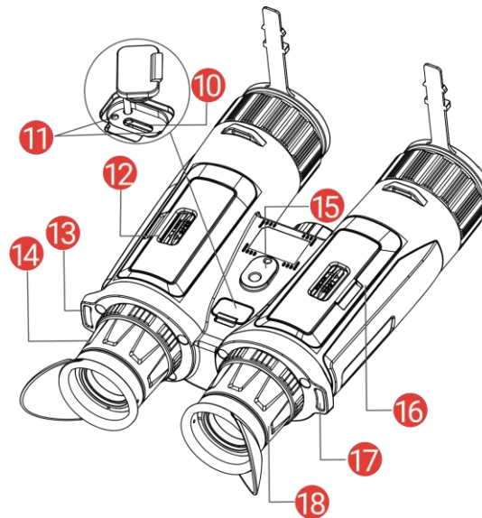
Abbildung 1-1 Aufbau
